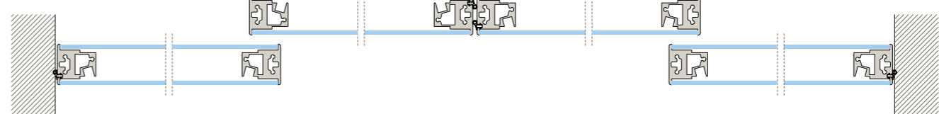
SEZIONE ORIZZONTALE
