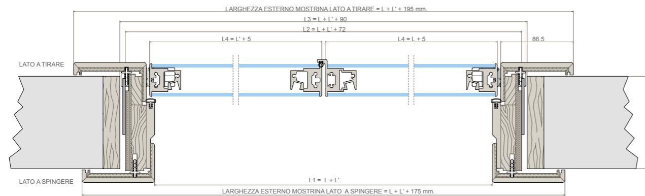
SEZIONE ORIZZONTALE
