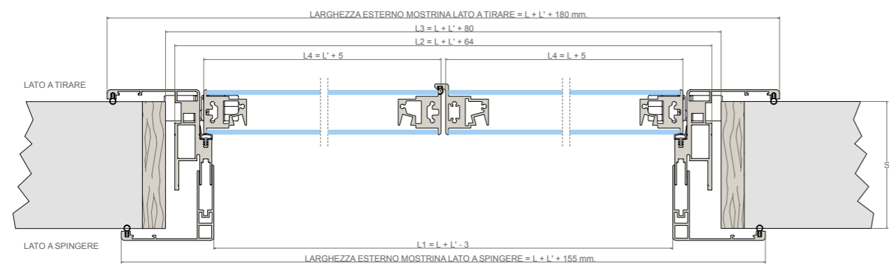
SEZIONE ORIZZONTALE
